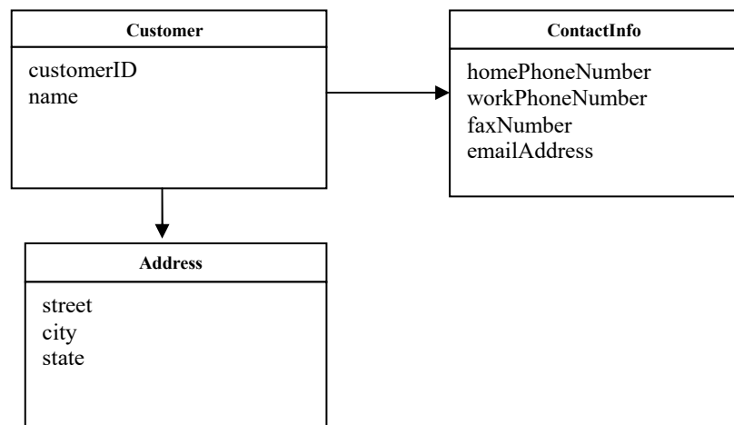
Рис. 3. Пример агрегата Customer
